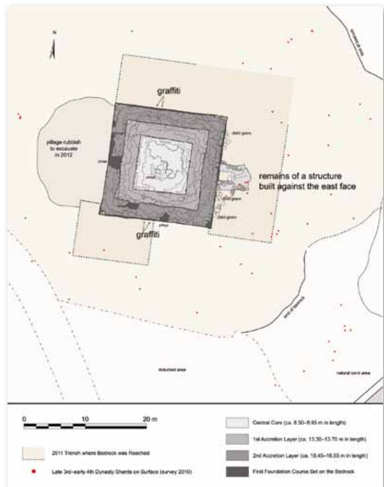
Fig. 5 Detaljeret plan af pyramiden i 2011.
